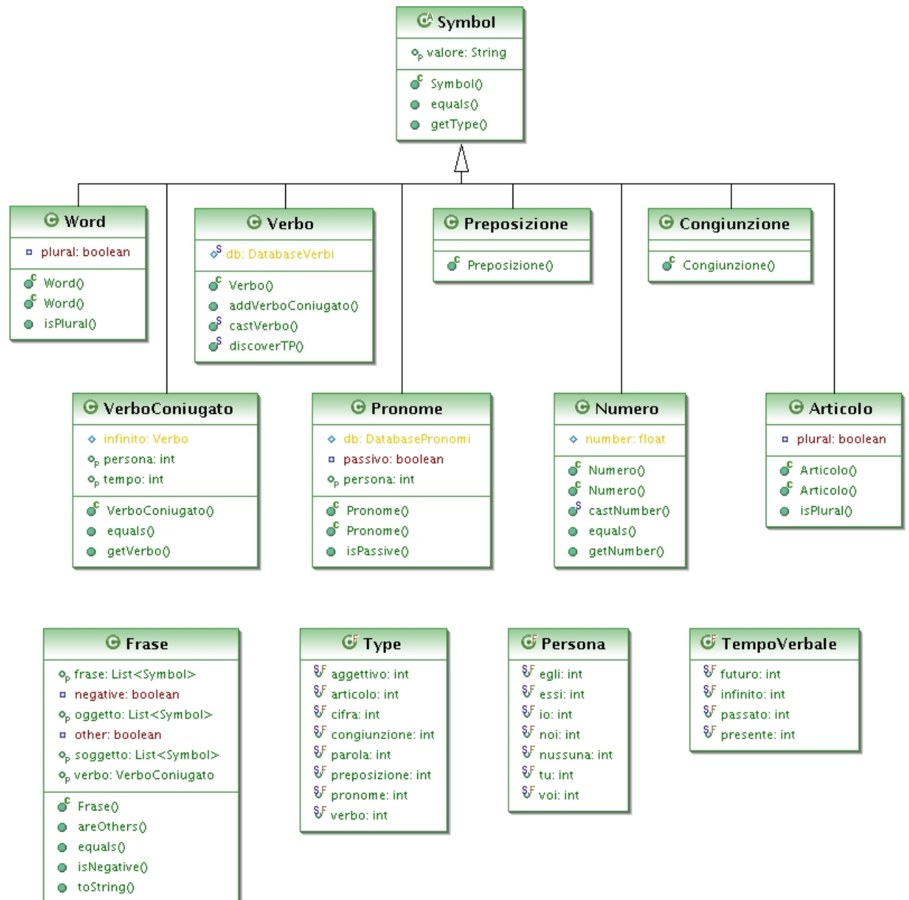
Figura 5.3: Schema UML del pacchetto types
