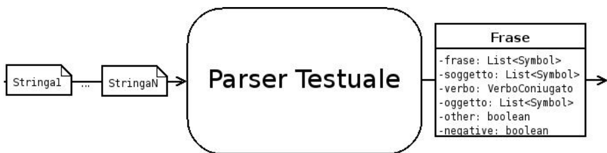
Figura 5.1: Schema del parser
