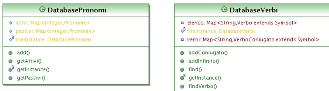
Figura 5.4: Schema UML del pacchetto databases
