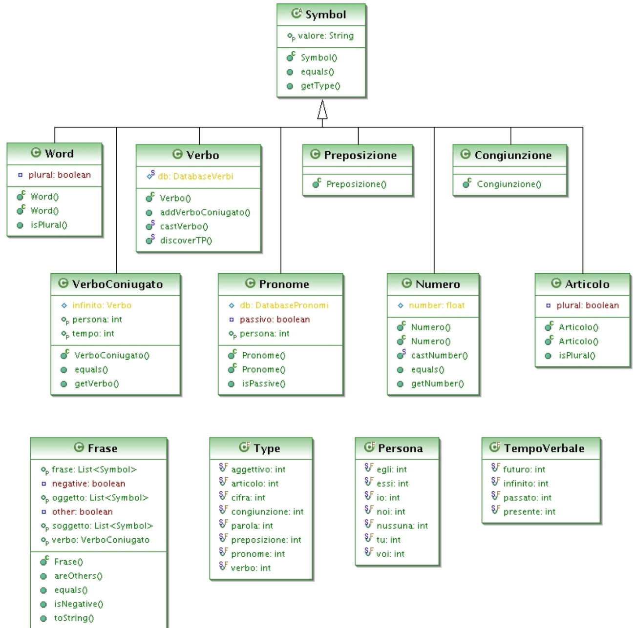
Figura 4.3: Schema UML del pacchetto types
