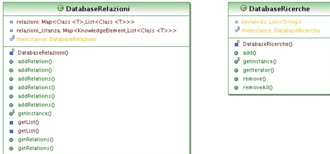
Figura 5.3: Schema UML del pacchetto databases
