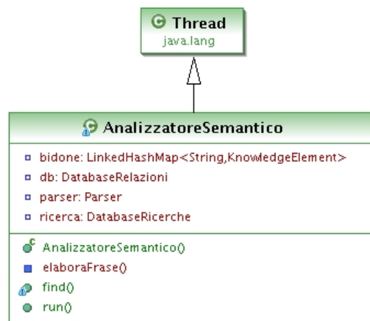
Figura 5.4: Schema UML della classe AnalizzatoreSemantico
