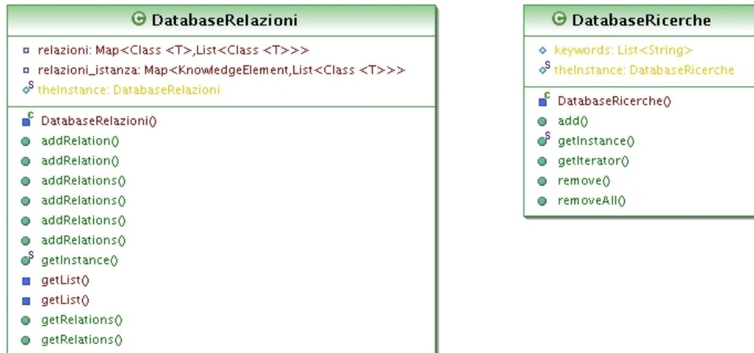
Figura 5.3: Schema UML del pacchetto databases
